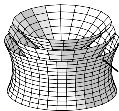
Niveauflächen der Funktion (x, y, z) \mapsto x^2 + y^2 - z^2
